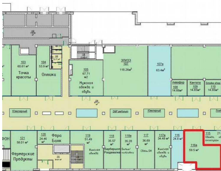
Схема планировки 1 этажа
